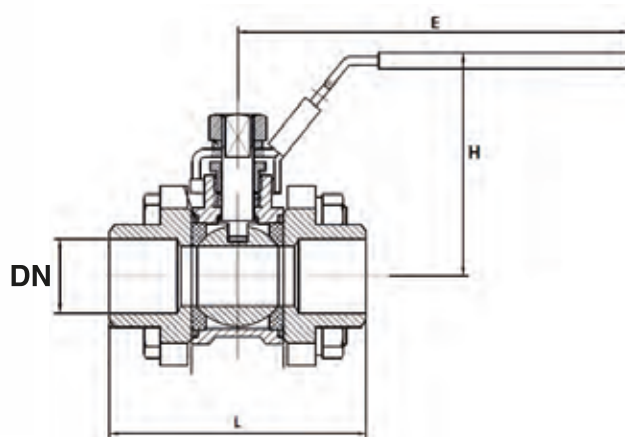
Dimensions Robinet 3 pièces (mm)
