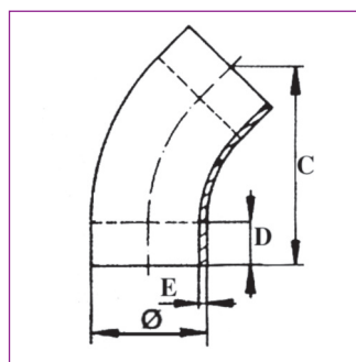
Coude 45° Elbows avec partie droite
