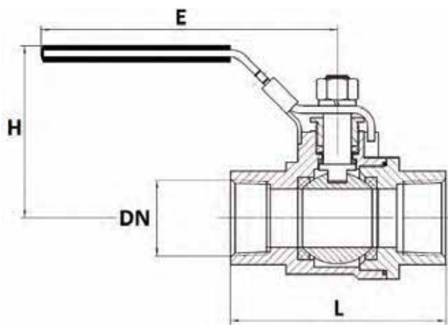
Dimensions Robinet 2 pièces (mm)
