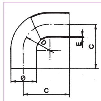
Coude 90° 3 D Elbows 90° 3 D avec partie droite
