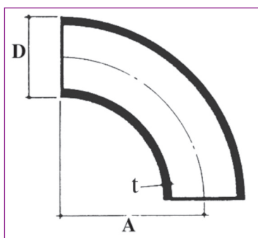
1,5 / 2 / 3 D 90° Métrique
