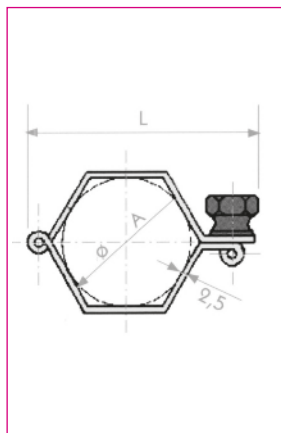
Collier à souder sans embase Type D
