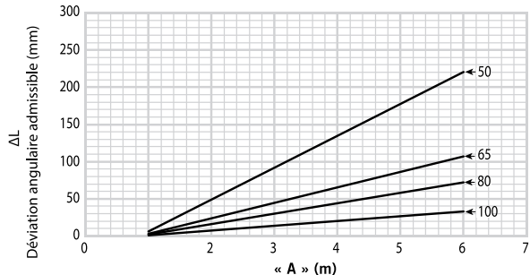
Mouvement StrengThin™ 100 – « paroi épaisse » 2 – 6"/DN50 – DN150 : Épaisseur du tube > 2,3 mm
