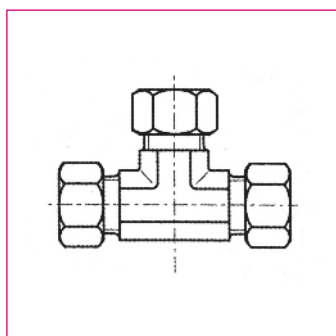
Té mâle
