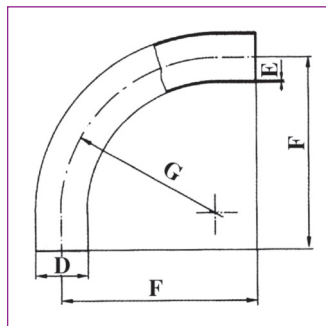
Coude 90° 1 D Elbows 90° 1 D avec partie droite
