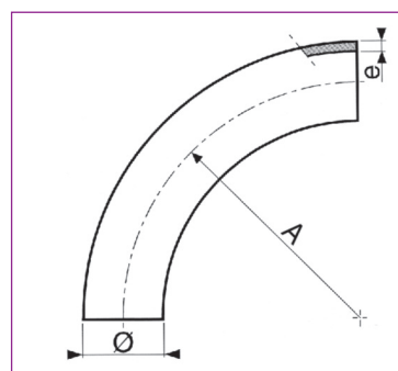
5 D 90° ISO
