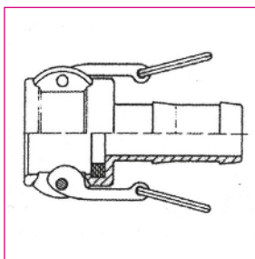
Coupleur cannelé
