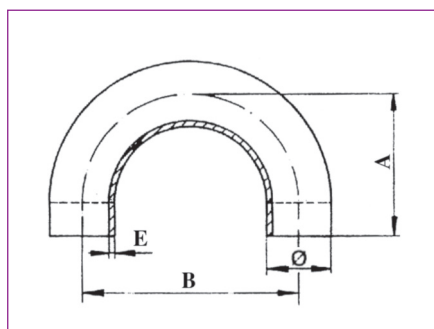
Coude 180° Elbows avec partie droite
