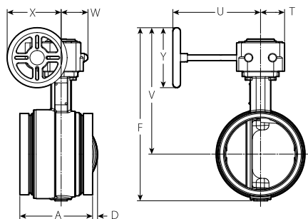
Vanne papillon – Volant réducteur 2 – 6"/DN50 – DN150
