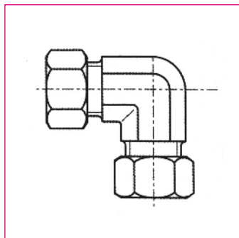
Coude égal
