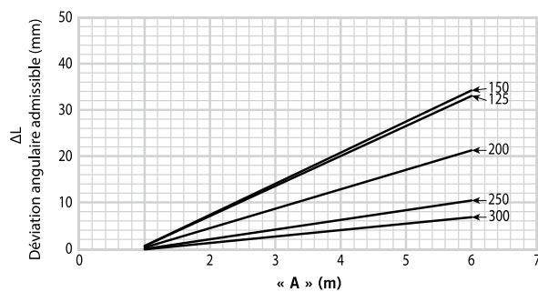
Mouvement StrengThin™ 100 – « paroi fine » 8 – 12"/DN200 – DN300 : Épaisseur du tube ≤ 3,1 mm
