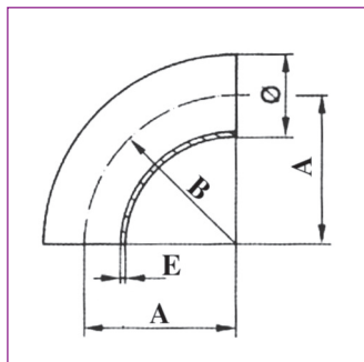
Coude 90° 1,5 D Elbows 90° 1,5 D sans partie droite
