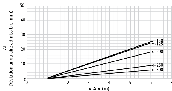
Mouvement StrengThin™ 100 – « paroi épaisse » 8 – 12"/DN200 – DN300 : Épaisseur du tube > 3,1 mm
