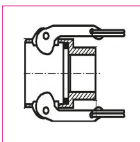
Coupleur à souder BW
