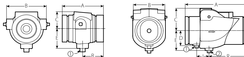
2 – 3"/DN50 – DN80 ① NPT ou vidange en aval BSPT (en option)
