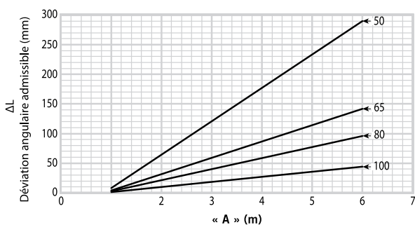
Mouvement StrengThin™ 100 – « paroi fine » 2 – 6"/DN50 – DN150 : Épaisseur du tube ≤ 2,3 mm
